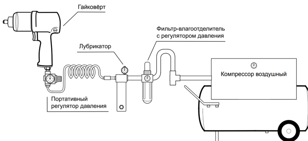
Рисунок 1. Схема воздушной магистрали
